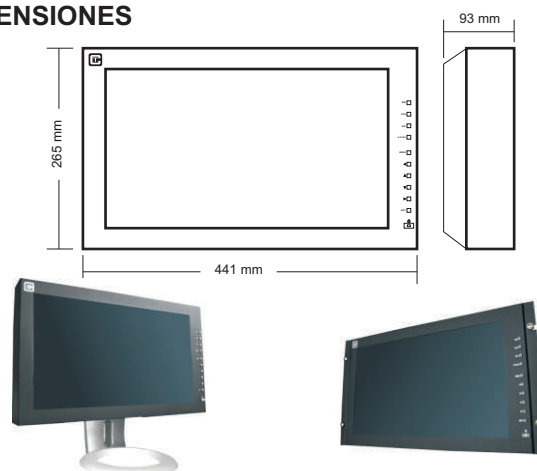
CA-PE15-17: Pie de sobremesa AC170WR: Kit montaje rack 19"
